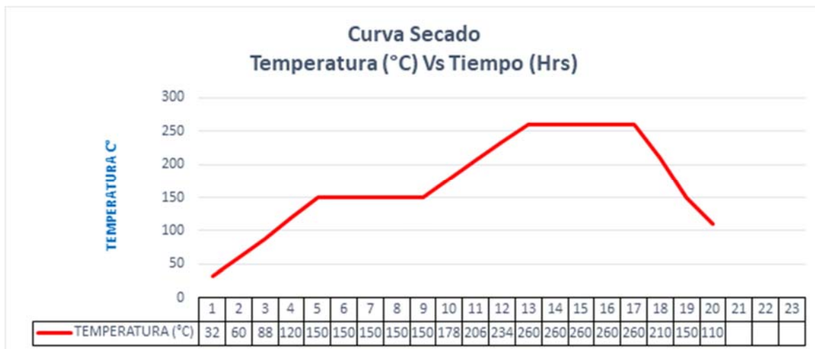
Figura 5. Curva de secado requerida
