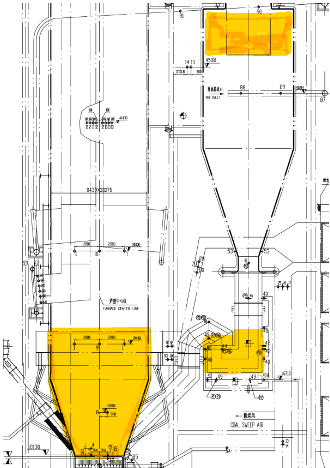
Figura 6. Vista lateral caldera. Zonas de posible reparación de refractarios
