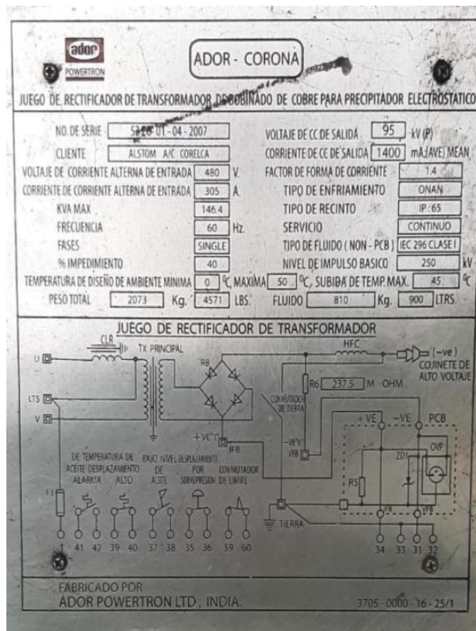
Datos de placa transformadores de campos precipitadores
