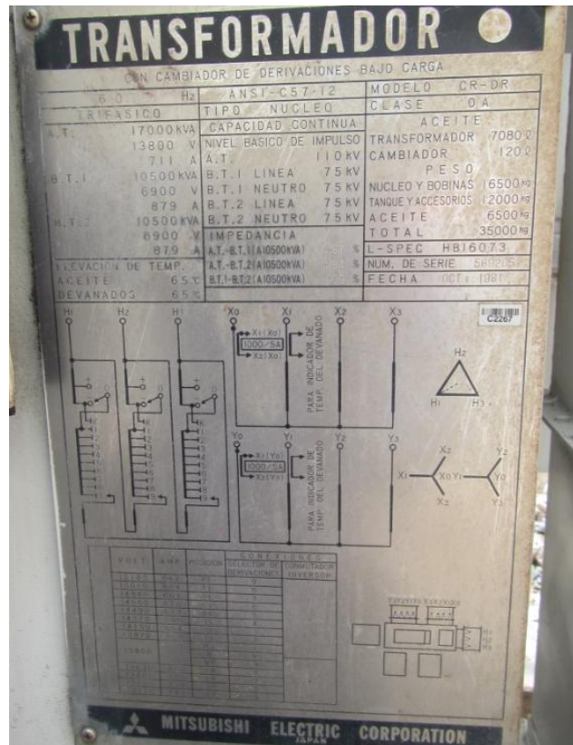
Datos de placa transformador auxiliar unidad No 1
